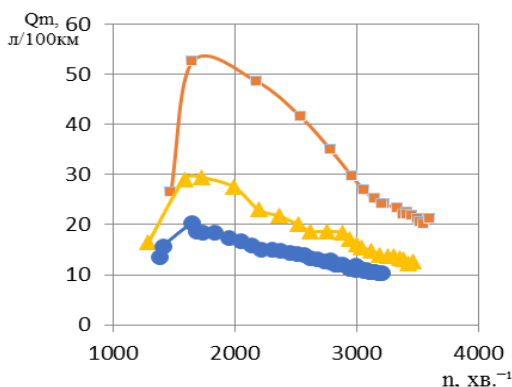
Рисунок 1 – Залежність миттєвої витрати палива автомобіля при навантаженні двигуна 10% на першій ■, другій ▲, третій ● передачах при температурі двигуна від -10 °С.
