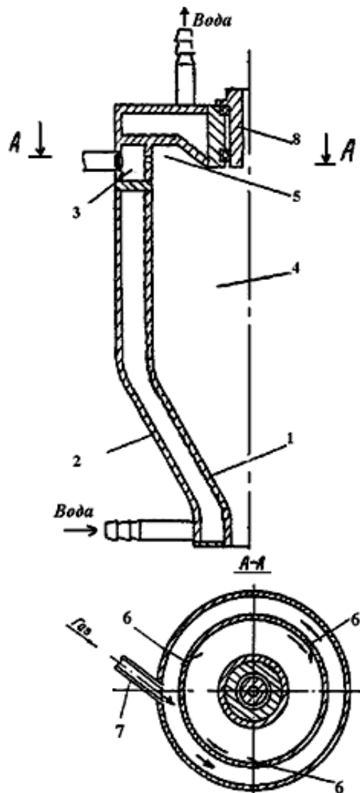
1 - труба переменного сечения; 2 - кожух; 3 - кольцевая полость; 4 - центральный канал; 5 - кольцевое углубление; 6 - боковые каналы
