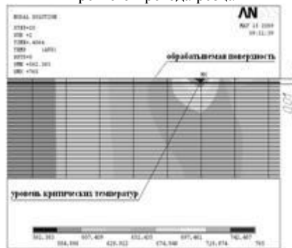
температурные поля заготовки в прирезцовой зоне после третьего прохода резца
