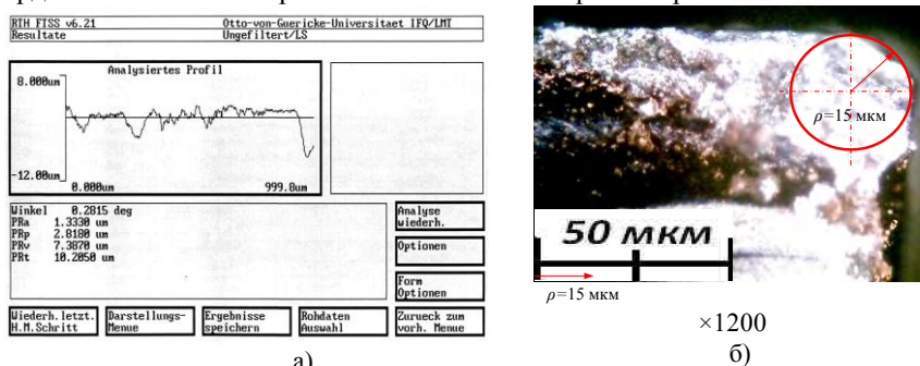
Рисунок 10 – Профилограмма шероховатости (а) и микрофотография радиуса округления (б) режущей кромки твердого сплава «ВолКар»
