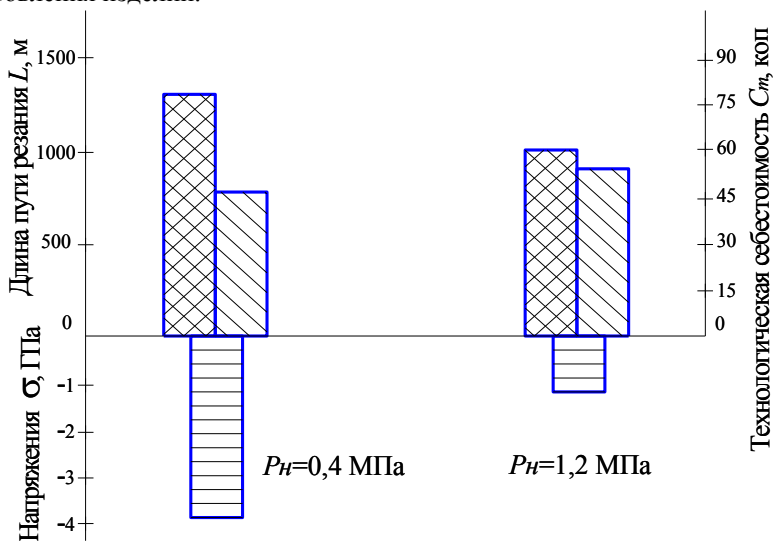
Рисунок 14 – Сравнительна диаграмма значений остаточных макронапряжений, длины пути резания и суммарной технологической себестоимости \sigma , L , C_m , круг 12A2-45° АС6 100/80 М1-01-4; V = 25 м/с; обрабатываемый материал «ВолКар»
