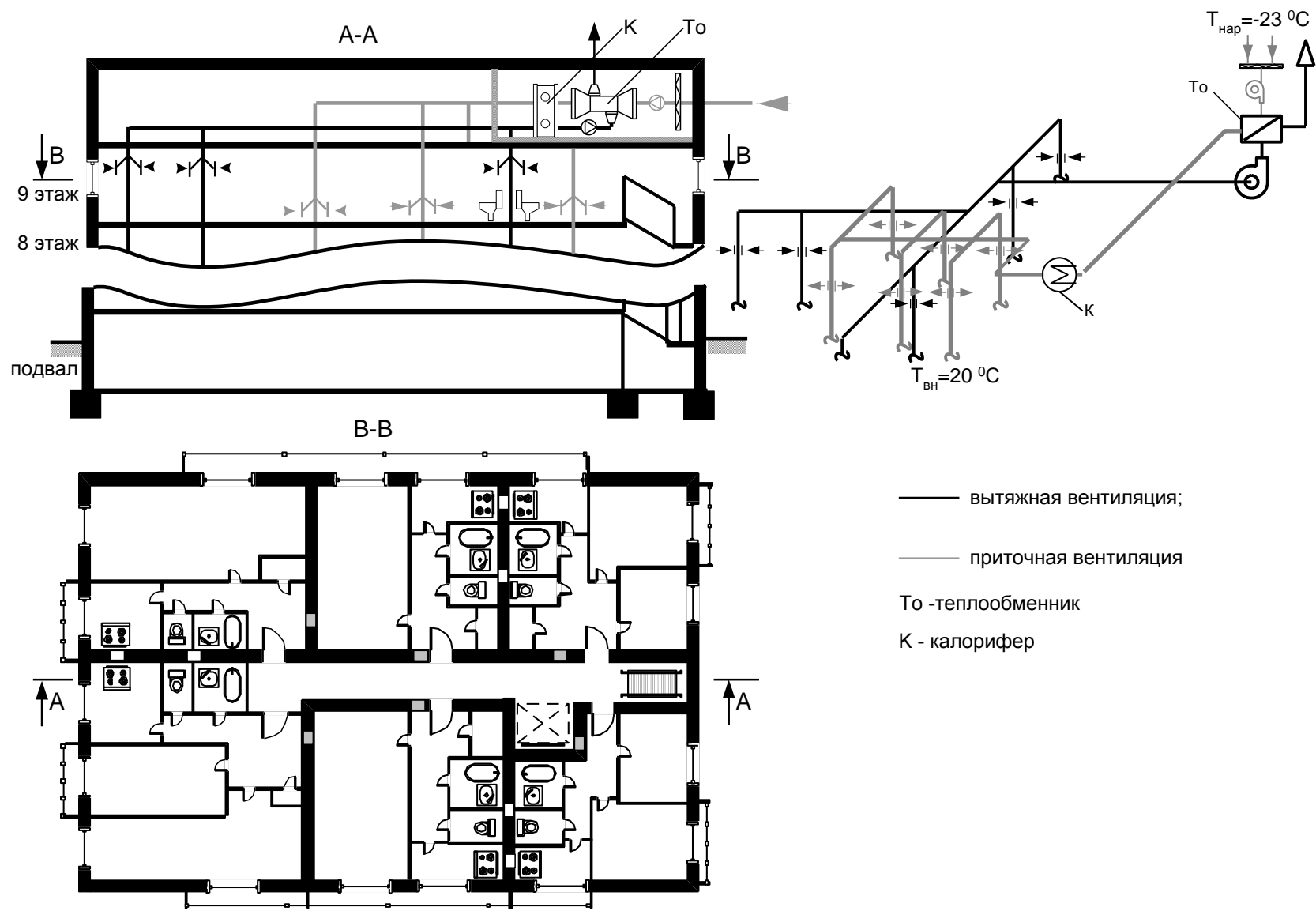
Рисунок 2 – Общая схема системы приточно-вытяжной вентиляции жилого здания типовой серии I-447 С-42
