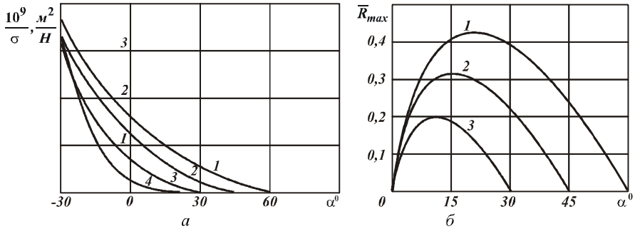
Рис. 2 – Залежність 1/\sigma (а) і \bar{R}_{\max} (б) від кута \alpha :
