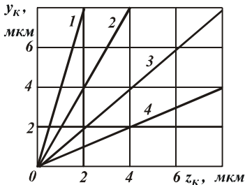
Рис. 4 – Функціональний зв'язок між координатами y_\kappa й z_\kappa зерна, що рухається:
