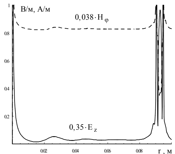
Рис. 2. Структура электромагнитного поля в сечении туловища человека на уровне двенадцатого позвонка в сторону живота
