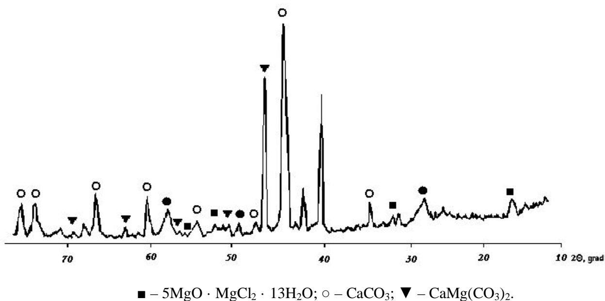
Рис. 3. Рентгенограма каустичного доломіту замішаного, бішофітом після 28 діб тверднення у воді
