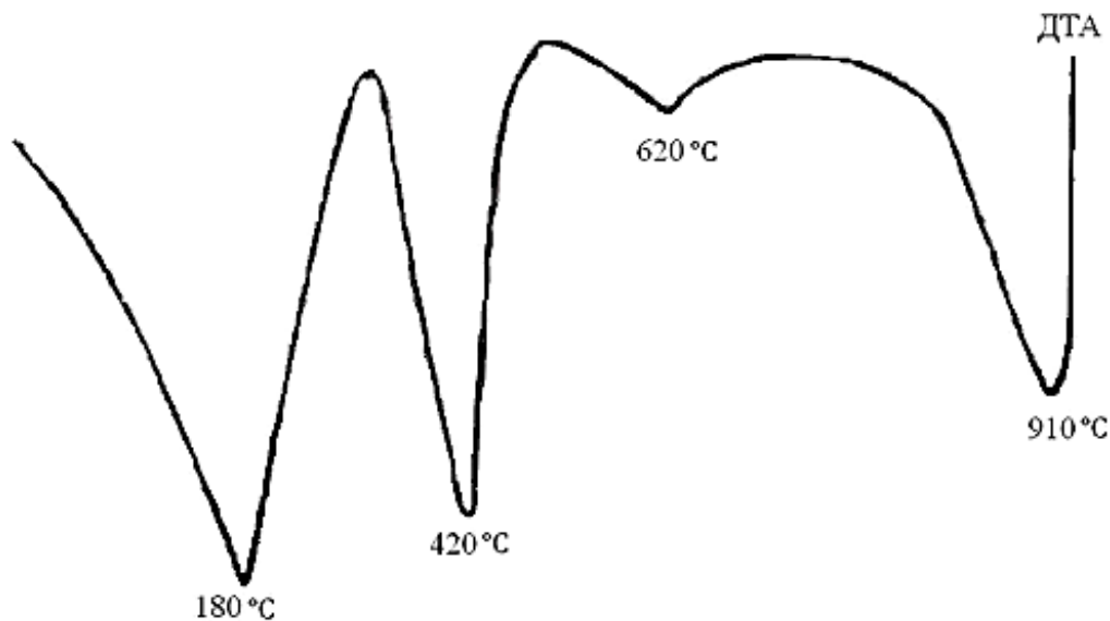
Рис. 2. Термограма каустичного доломіту замішаного, бішофітом після 28 діб повітряного тверднення
