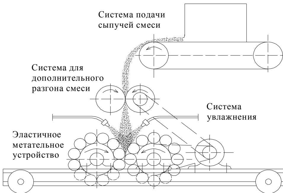
Рис. 1. Схема агрегата формирования тонкостенных конструкций
