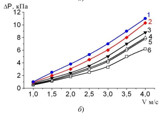
Рисунок 1 – Залежність гідравлічного опору шару катализатора для зерна різної форми та розмірів: а) від висоти шару ( h ), w = 3 м/с: 1 – 5:0:20; 2 – 10:4:20; 3 – 7:2,5:20; 4 – 6:2:20; 5 – 5:2:20; 6 – 4:1,5:20; 7 – 5:0:5; б) від лінійної швидкості: 1 – 5:0:20; 2 – 10:4:20; 3 – 7:2,5:20; 4 – 6:2:20; 5 – 5:2:20; 6 – 4:1,5:20; 7 – 5:0:5
