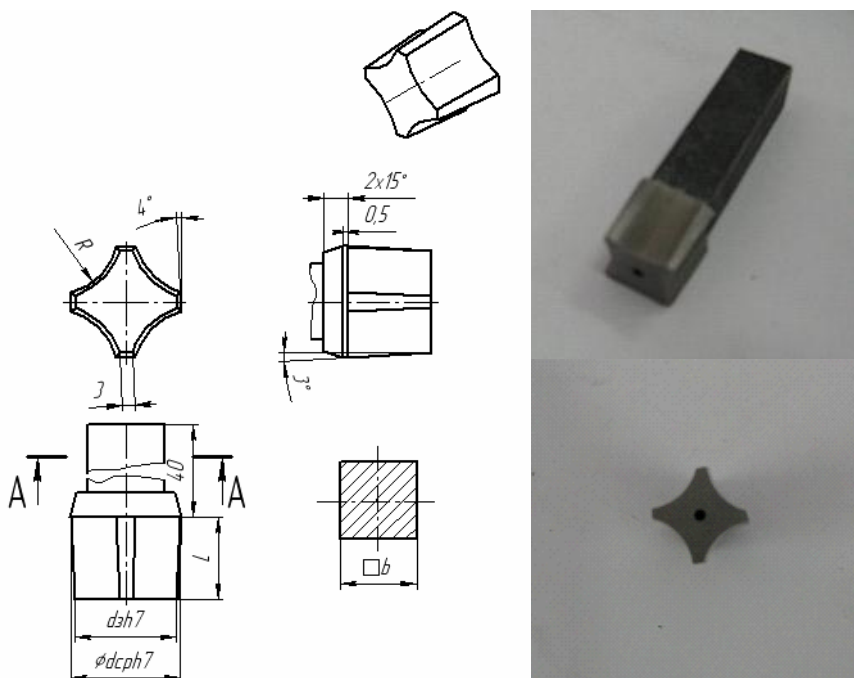
Рисунок 3 – Деформирующий инструмент для глухих отверстий
