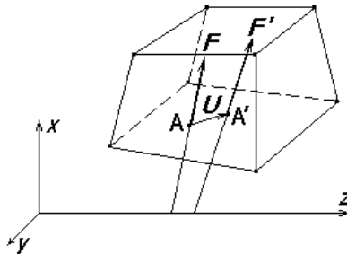
Изменение центробежной силы при смещении точки КЭ
