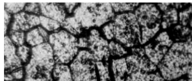
Рис. 2. Мікроструктура фольги Та (x450) чистотою 99,99 % після відпалу 1000 °С (1 година).
