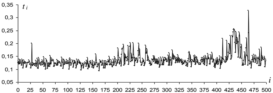
Рис. 1. Замеры времени выполнения (сек) периодически вызываемой программы в многозадачной среде Windows (500 измерений)
