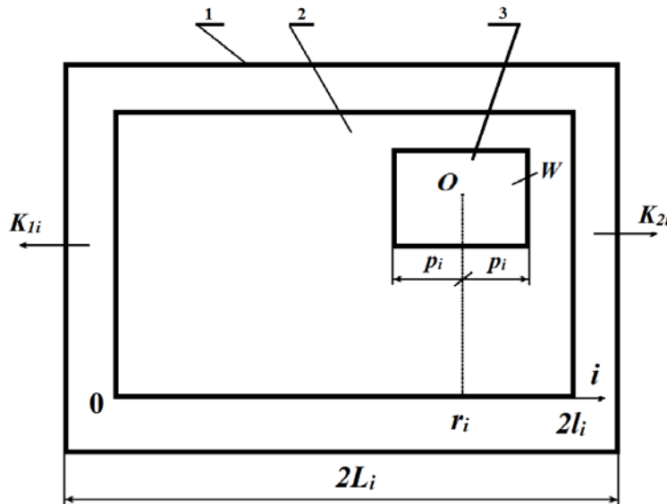
Рис. 1. Тепловая модель формы параллелепипеда с источником тепла:
