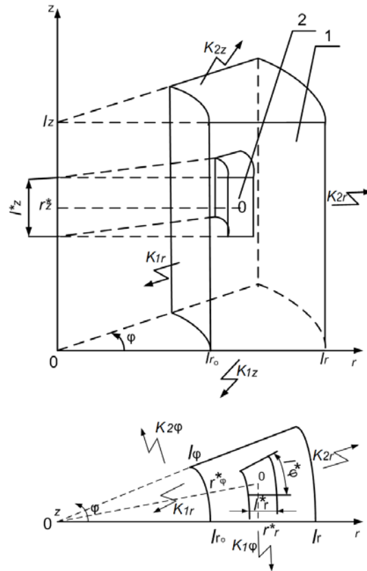
Рис. 2. Тепловая модель нагретой зоны с источником тепла, имеющих форму цилиндра, ограниченного координатными поверхностями: 1 – нагретая зона; 2 – источник тепла
