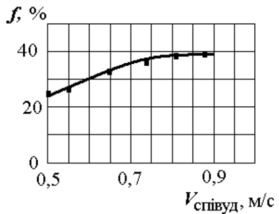
Рисунок 14 – Зміна коефіцієнта розкриття мінералів від швидкості співудару молольних тіл
