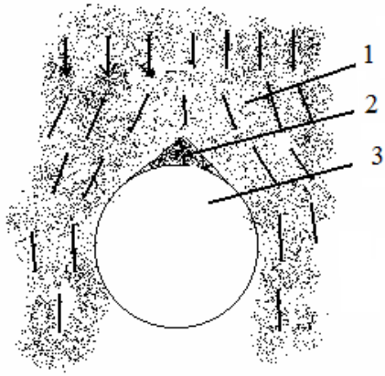
Рисунок 5 – Схема обтікання кулі потоком сипкого середовища: 1 – сипке середовище; 2 – приєднаний конус; 3 – молярне тіло (куля).
