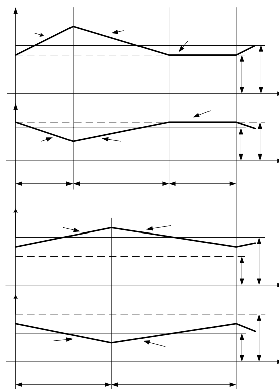
Рис. 2. Диаграммы токов двигателя при а) «легком» ослаблении возбуждения, t_M \neq 0 ; б) «глубоком» ослаблении возбуждения, t_M = 0 .
