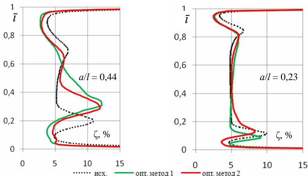
Рис. 4. Распределение коэффициента потерь по высоте на выходе из решетки
