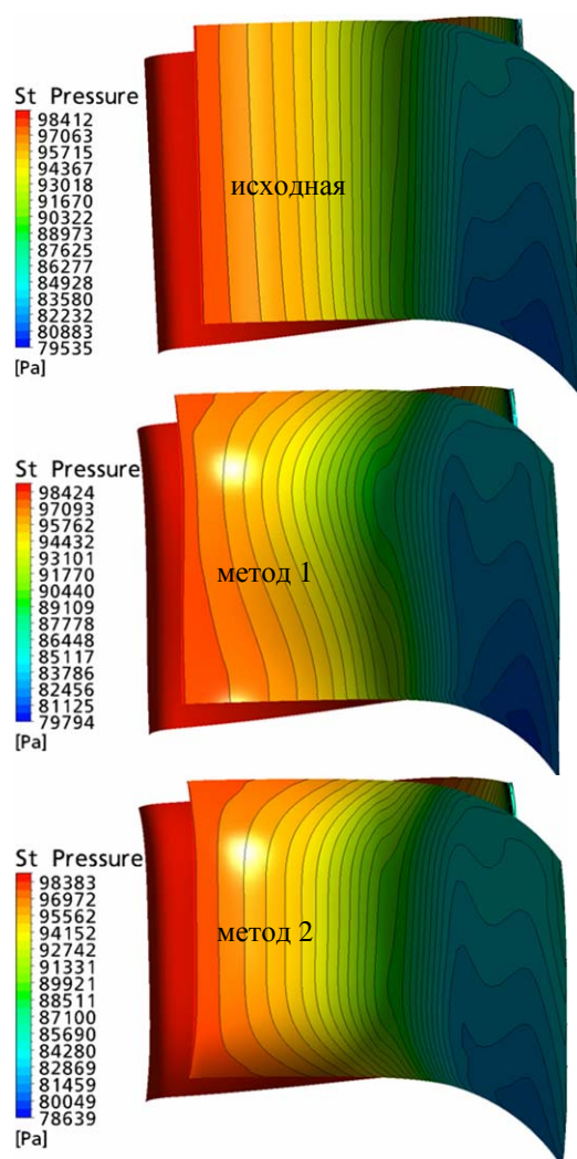
Рис. 7. Поле статического давления на спинке лопатки при a/l = 0,23
