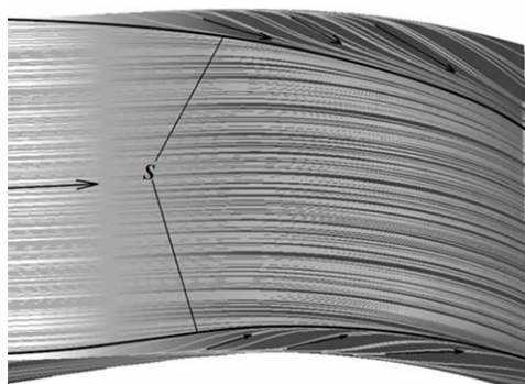
Рис. 6. Линии тока на спинке исходной лопатки
