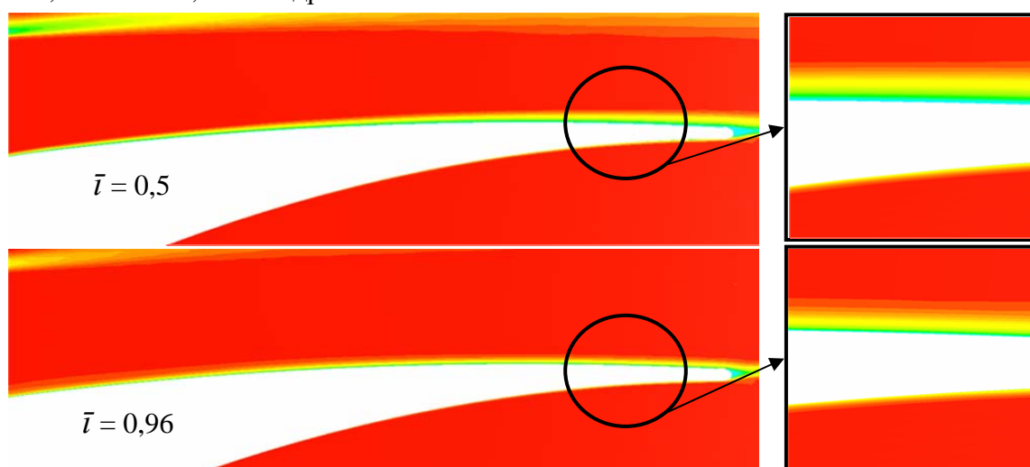
Рис. 5. Поле полного давления в исходной решетке
