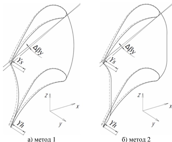
Рис. 2. Параметрическая форма турбинной лопатки
