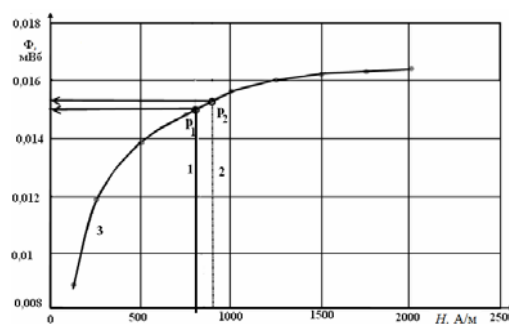
Рис. 1. Зависимость магнитного потока от напряженности магнитного поля
