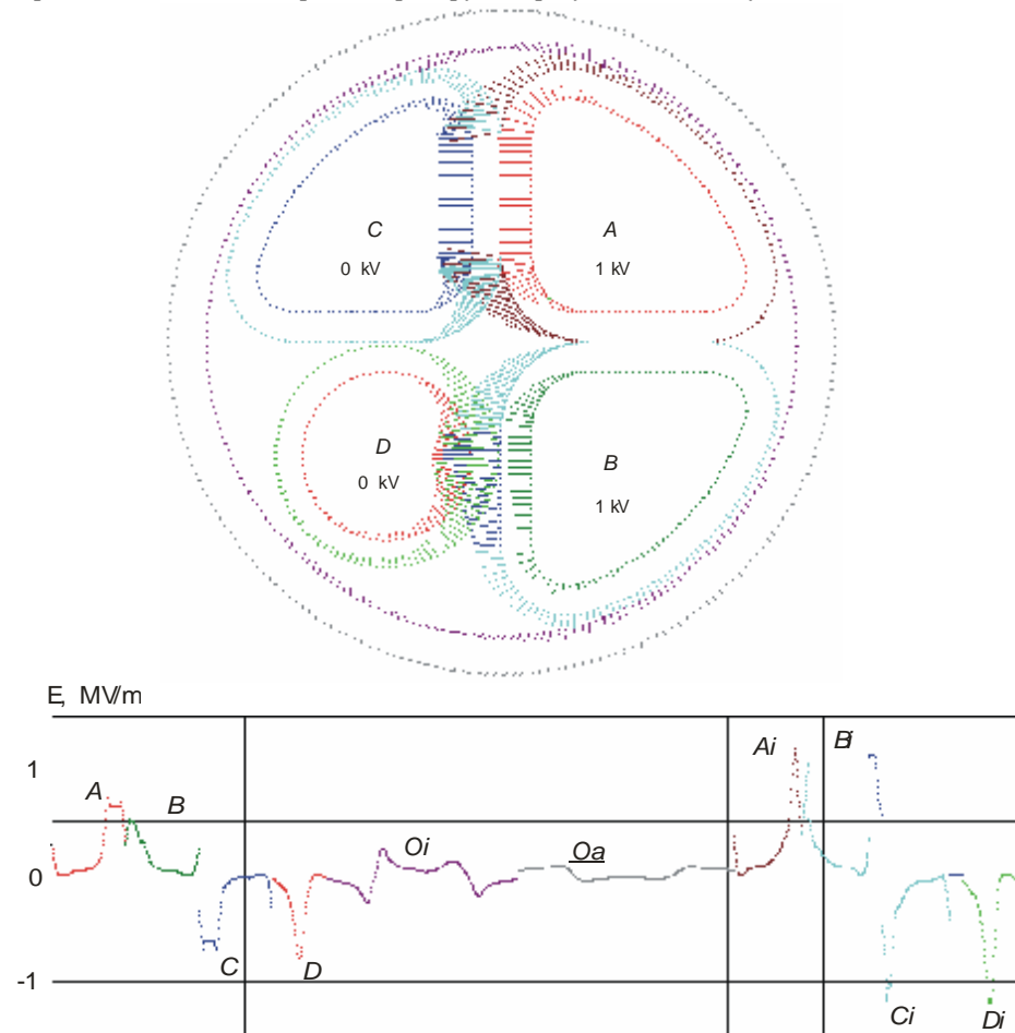
Рис 1 - Дипольное распределение потенциала. Порядок расположения узлов: фазы А, В, С, D; затем внутренняя и внешняя поверхности оболочки; затем поверхности изоляции фаз
