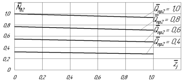
Рисунок 4 – Зависимость безразмерной мощности потока дополнительного расхода воздуха от безразмерной координаты его подвода в подъемную трубу \bar{N}_{в2} = f(\bar{z}_j) (базисные значения z_j = z_{jмакс} = 3,14 м, N_{в2} = 22,4 кВт, Q_{вп2} = 0,0222 м 3 /с)
