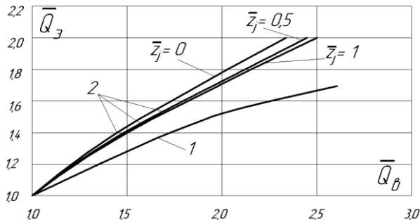
Рисунок 3 – Безразмерные расходные характеристики эрлифта \bar{Q}_3 = f(\bar{Q}_B) традиционной 1 и предлагаемой 2 схем при разных значениях z_j (базисные значения z_j = z_{jмакс} = 3,14 м; Q_3 = 0,0222 м 3 /с; Q_B = 0,273 м 3 /с)
