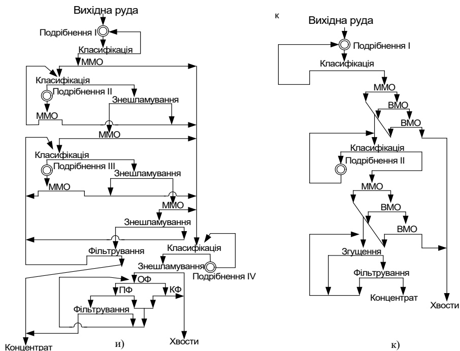
Рисунок 4 – Принципові технологічні схеми збагачення тонковкраплених залізних руд: и – магнітно-флотатійна схема з 4-х стадіальним подрібненням, к – магнітна із збагаченням у сильному магнітному полі
