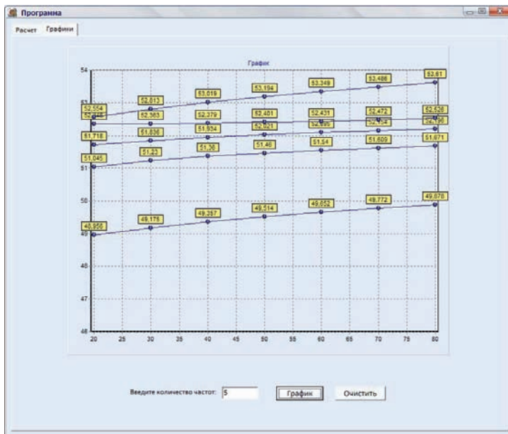
Рисунок 3 – Графики зависимости собственных частот от толщины стенки
