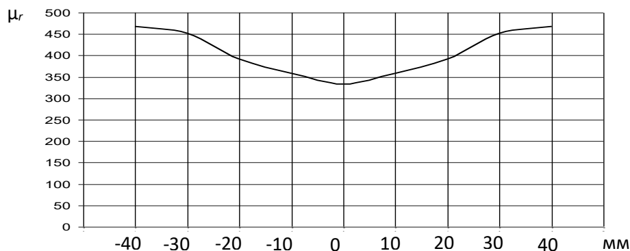
Рис. 3 – Зміна \mu_r в залежності від відстані до зварного шва з обох сторін
