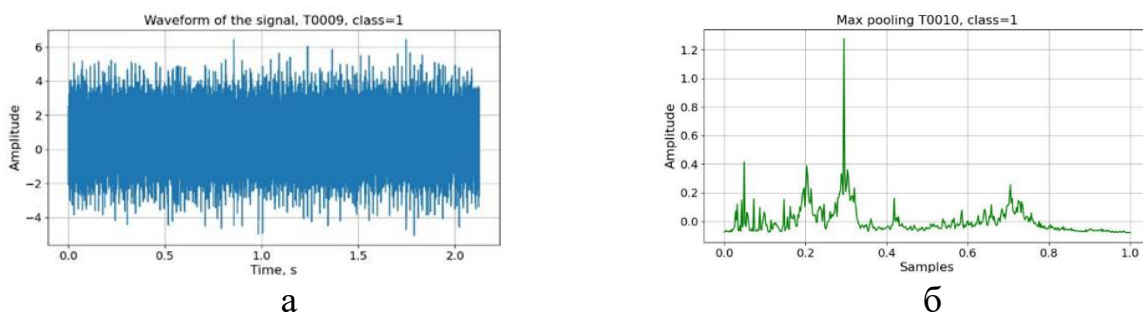
Рис 2 – Приклади обробленого вектора вхідних даних, який подається на вхід неймережі (а – вектор вібрацій механізмів з повністю робочого гвинтокрила до обробки, б – та після)
