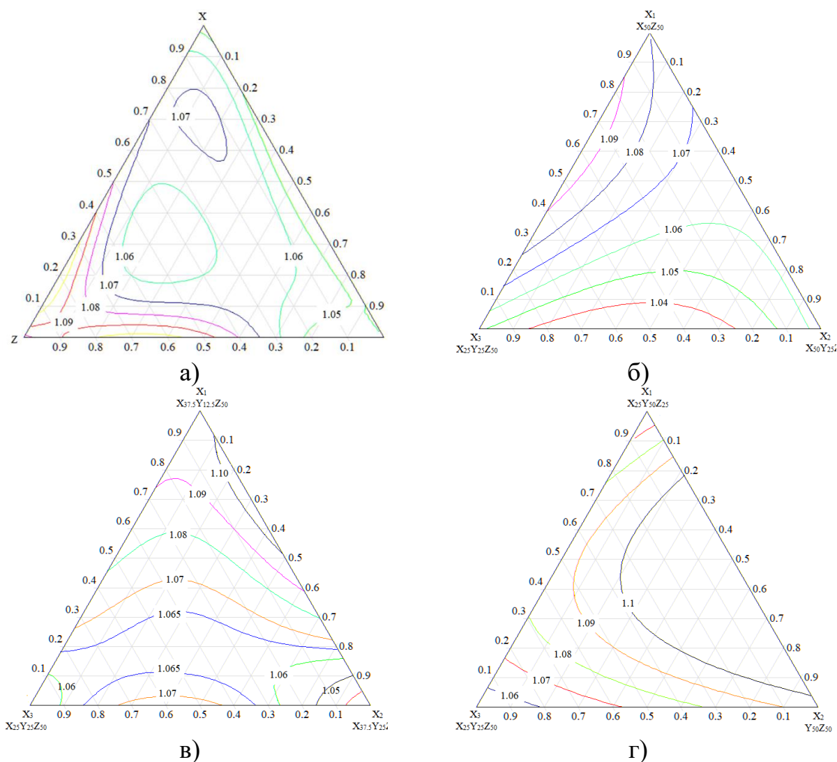
Рис. 1 – Ізолії значень коефіцієнта ущільнення для досліджуваних складів шихт
