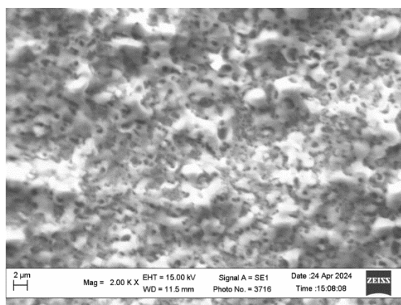
Рис. 2 – Мікроскопія поверхні покриття
