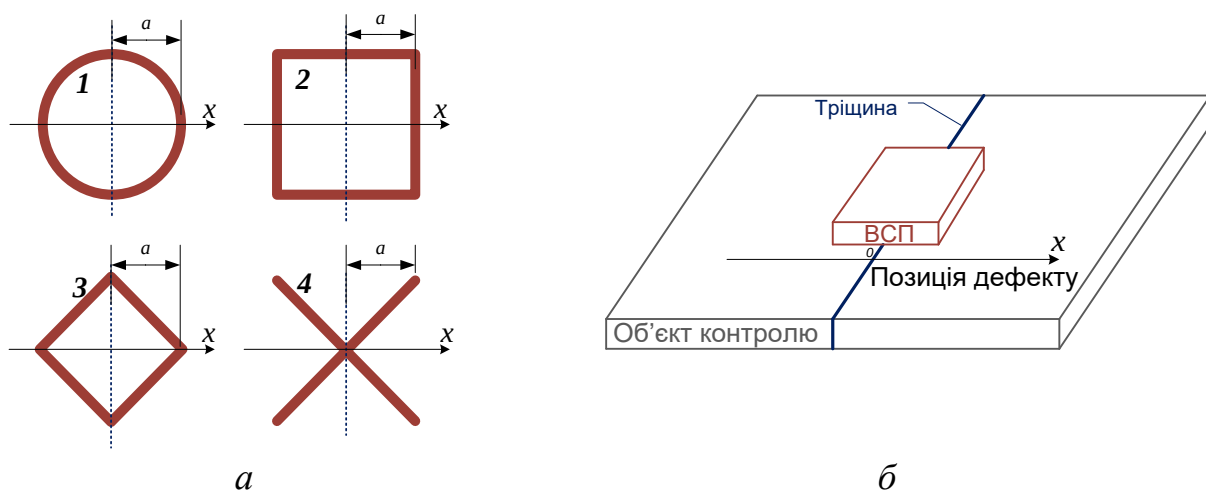
Рис. 1 – Дослідження впливу позиції дефекту для ВСП з різними обмотками: а – конфігурації обмоток ВСП; б – моделювання впливу позиції дефекту
