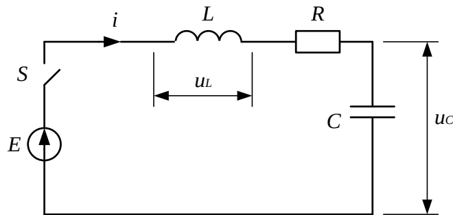
Рис.3 – Схема заміщення ПД-регулятора приводу запуску дрона
