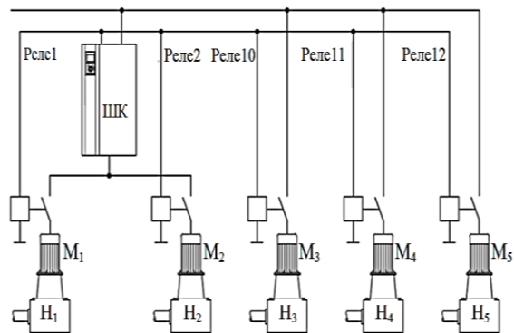
Рис. 2 – Змішана конфігурація насосів
