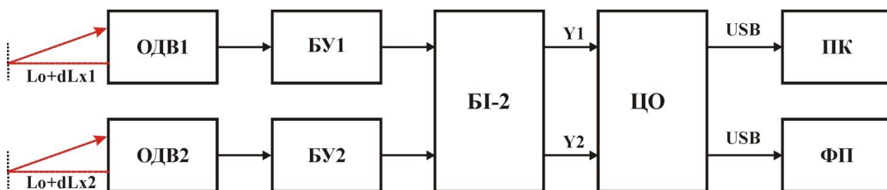
Рис. 1 – Функціональна схема системи вимірювань
