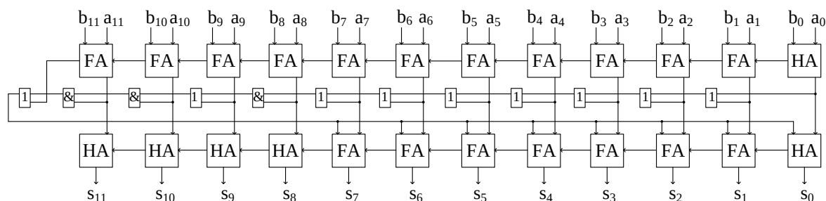
Рис. 1 – Структурна схема суматора для модуля P = 3329
