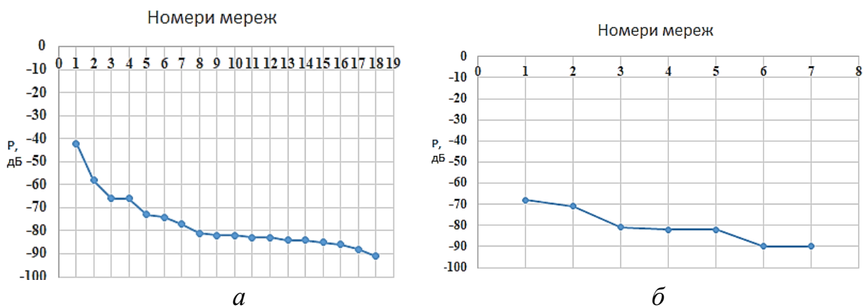
Рис. 1 – Графіки потужностей сигналу мереж Wi-Fi: а – з антеною; б – без антени
