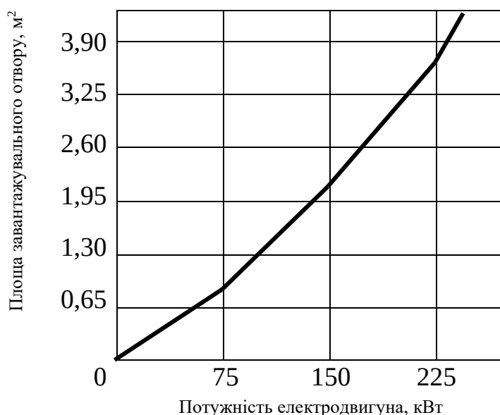
Рис. 2 – Залежність установчої потужності електродвигуна від площі завантажувального отвору дробарки
