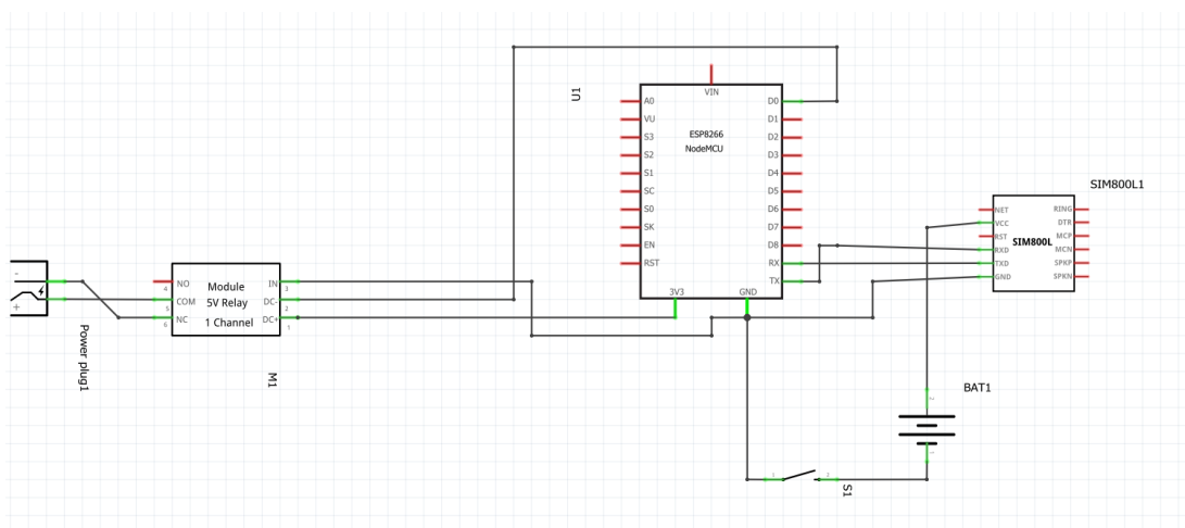
Рис. 1.1– Електрична схема підключення пристрою сповіщення
