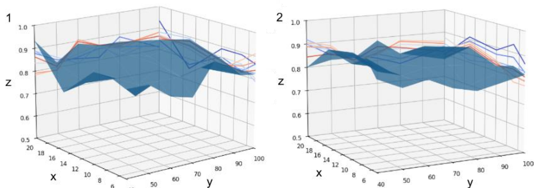
Рис. 1 – Аналіз впливу періодів попереднього навчання з використанням EEG дорослих (x) і навчання (y) з використанням EEG немовлят на точність моделі (z) Shallow ConvNet для 700 (1) та 1200 (2) сигналів, використаних для попереднього навчання
