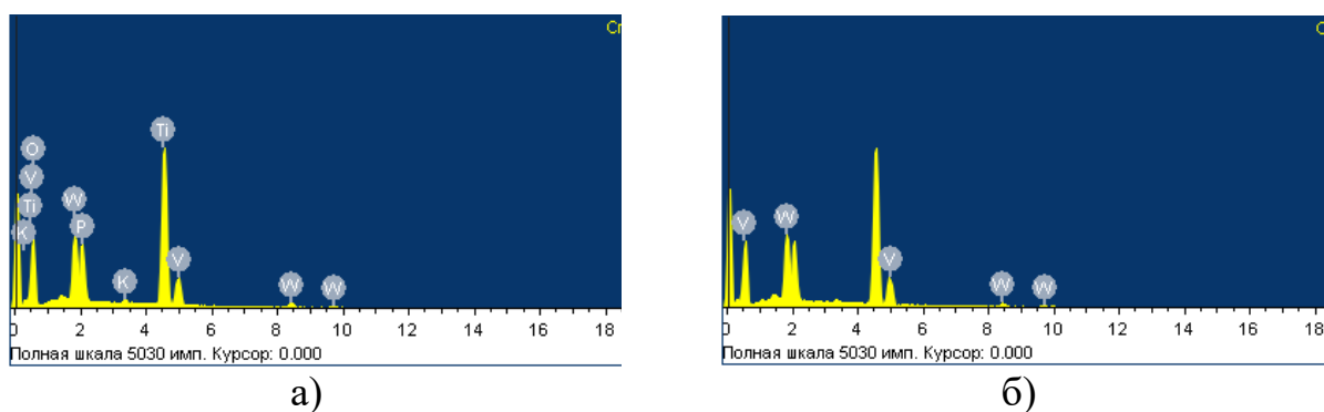
Рис. 1 – Результати визначення елементного складу покриття: а – поверхня (ат. %: Ti-27,59; O-60,99; P-6,76; K-0,32; V-1,51; W-2,83); б – виступи сфероїдів (ат. %: V-66,52; W-33,48)
