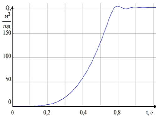
Рис. 3 – Перехідний процес Q(t) відцентрового насосу
