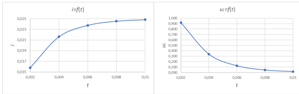
Рис.2 – Перехідні характеристики для П-регулятора
