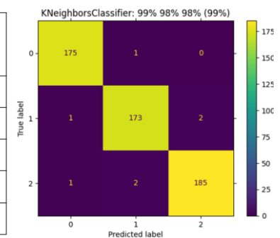
Рис.2 – а) Порівняння результатів класифікації; б) Матриця невідповідності для моделі на основі методу k найближчих сусідів (0-нормальний, 1-передіктальний, 2-іктальний стан)
