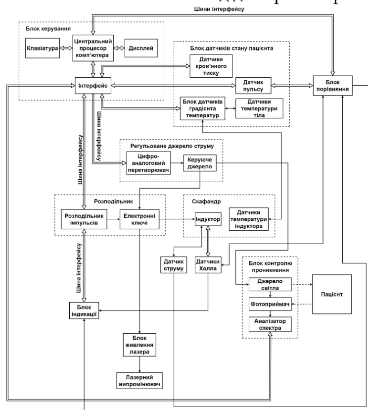
Рис. 1 – Схема комп'ютерно-інтегрованого комбінованого магнітотерапевтичного апарату
