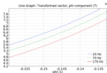
Рисунок 2 – графік залежності V_\phi від кутової координати \phi для струму 5А, частот 20, 70, 170 Гц, та радіусу 25.5 мм.
