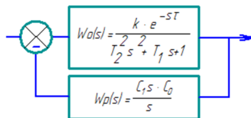
Рис. 1 – Структурна схема АСР
