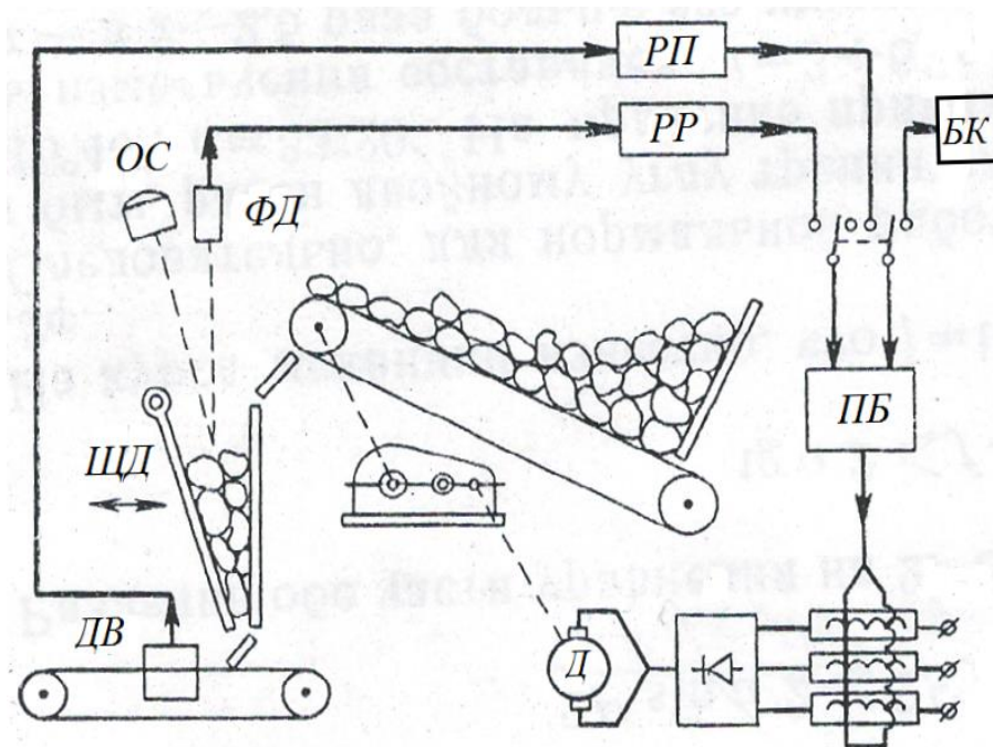
Рис. 1 – Блок-схема автоматичного регулювання завантаження щоківі дробарки
