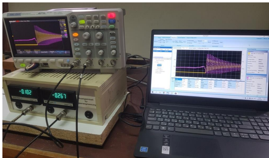
Рис.2 – Зовнішній вигляд системи індикації результатів вимірювань.
