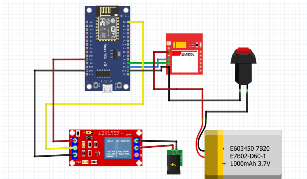
Рис. 1.2 – Макет приладу сповіщення
