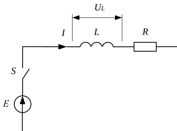
Рис.1 – Схема заміщення П-регулятора приводу запуску дрона
