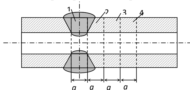
Рис. 1 – Ескіз фрагмента труби зі зварним швом та навколо шовною зоною
