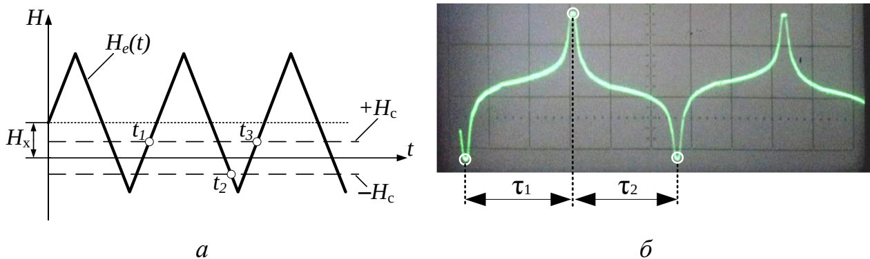
Рис. 1 – Часові діаграми сигналів фазоімпульсного ферозонда: a – сигнал збудження ферозонду; б – осцилограма вихідного сигналу з характерними точками
