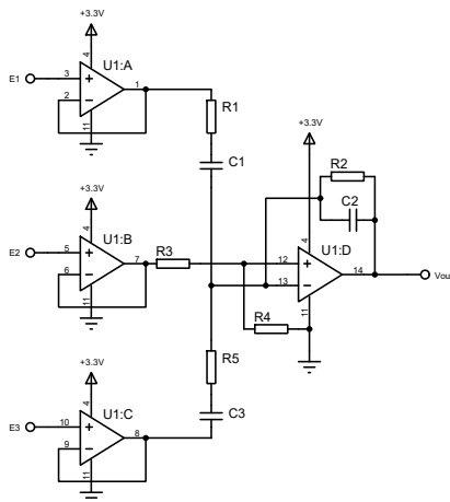
Рис.3 – Вузол зняття міосигналів
