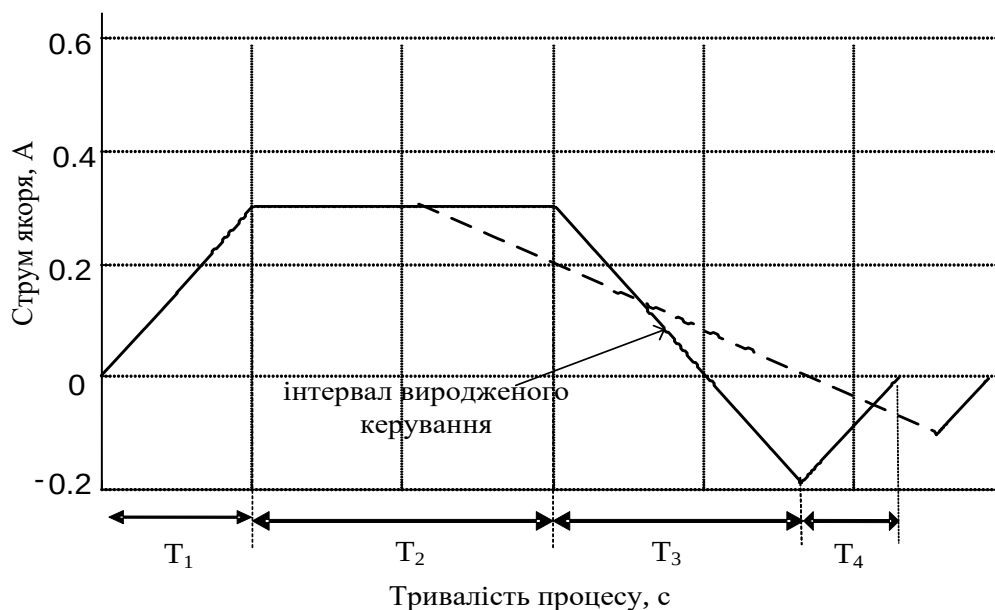
Рис. 1 – Процес енергозберігаючого керування
