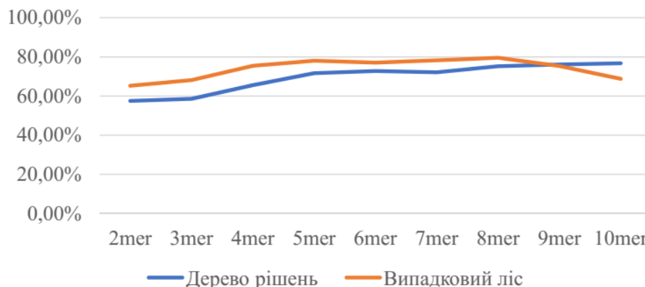
Рис.2 – Точність класифікації на 4 класи в залежності від довжини k -мерів
