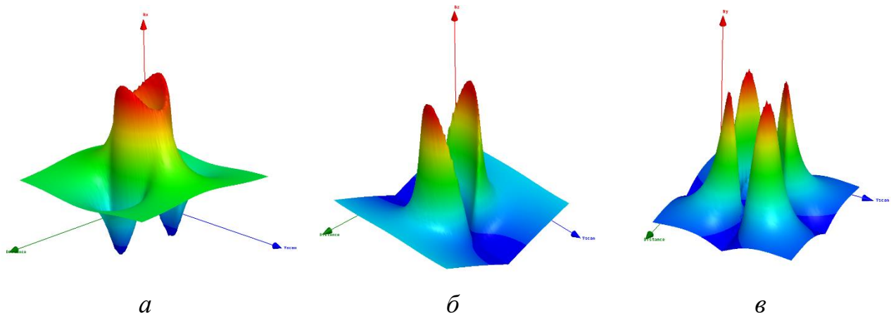
Рис. 2 – Розподіл складових магнітного поля округлого дефекту (амплітудні значення): а – B_x ; б – B_z ; в – B_y
