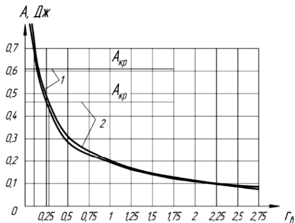
Рис. 1 – Графіки питомої роботи деформування в залежності від відносного внутрішнього радіусу згинання: 1 – для сталі Ст.3сп; 2 – для сталі 09Г2
