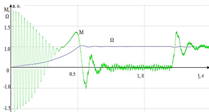
Рис. 4 – Пуск системи ПЧ – АД з накидом навантаження
