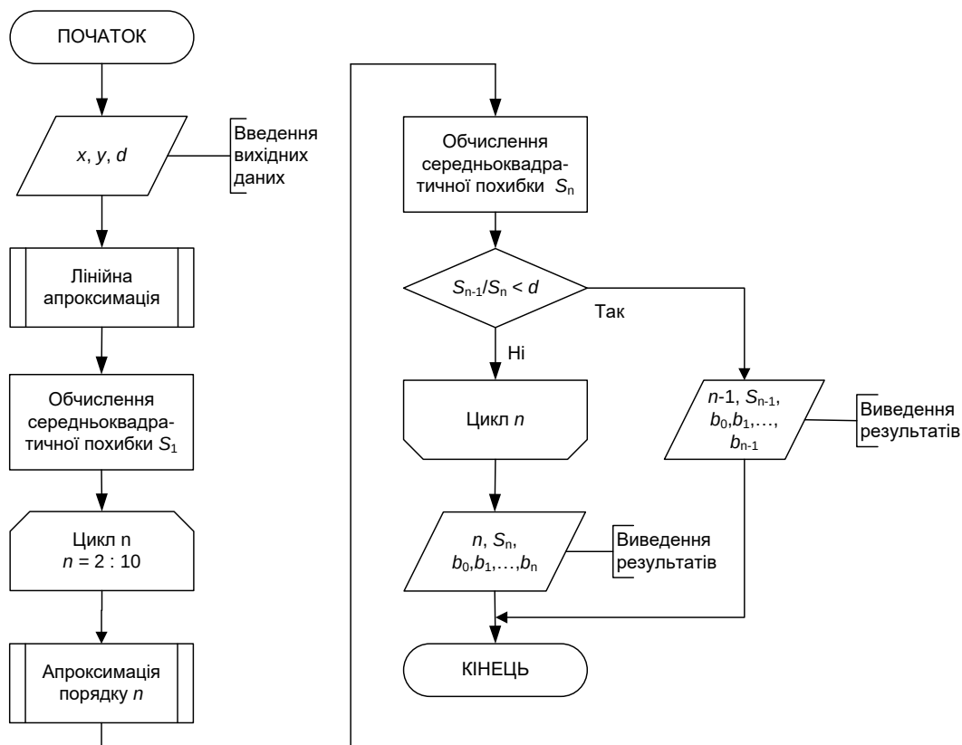
Рис. 1 – Алгоритм автоматизованого вибору порядку поліноміальної моделі
