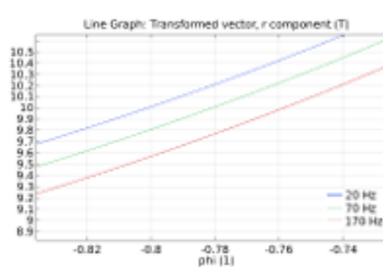
Рисунок 5 – графік залежності V_r від кутової координати \phi для струму 5А, частот 20, 70, 170 Гц, та радіусу 27 мм.
