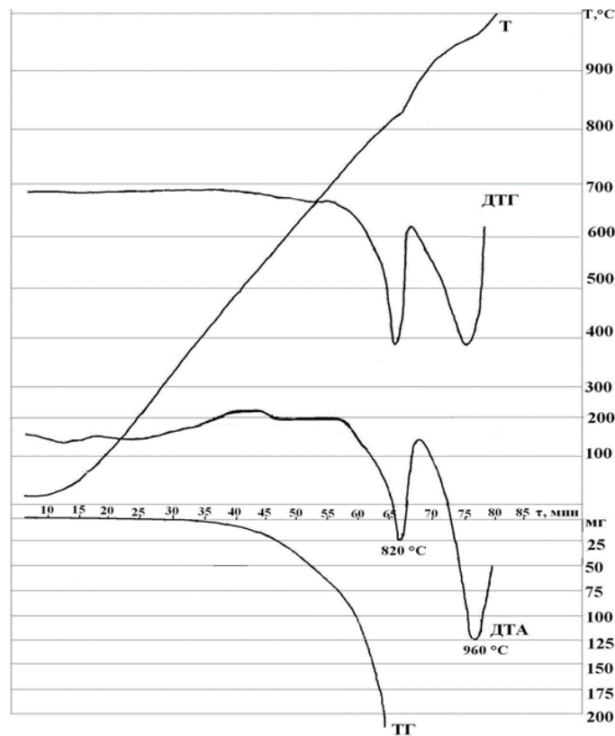
Рис. 1 – Дериватограма доломіту
