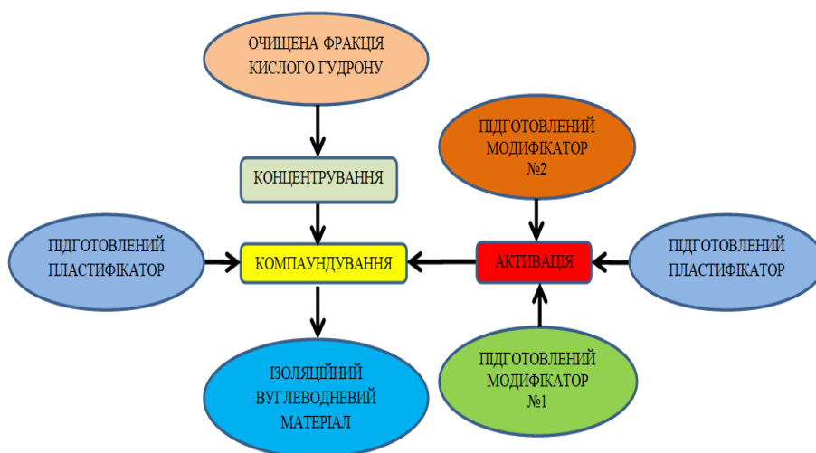
Рис. 1 – Схема виробництва ІВМ
