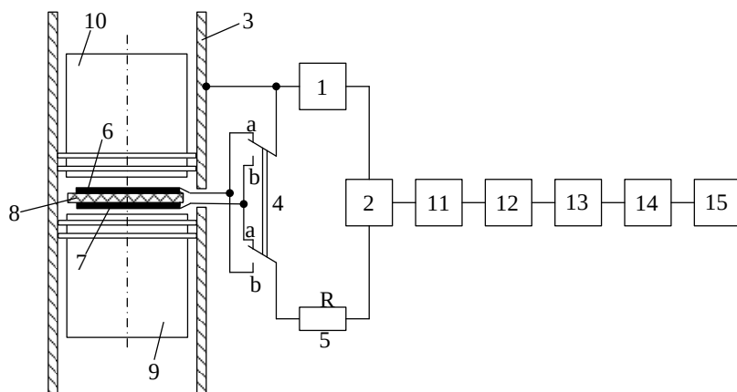
Рис. 1 – Блок-схема пристрою для визначення ВМТ в циліндрах дизеля
