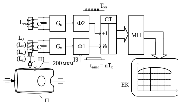
Рис. 1 – Структурна схема профілометра поршню
