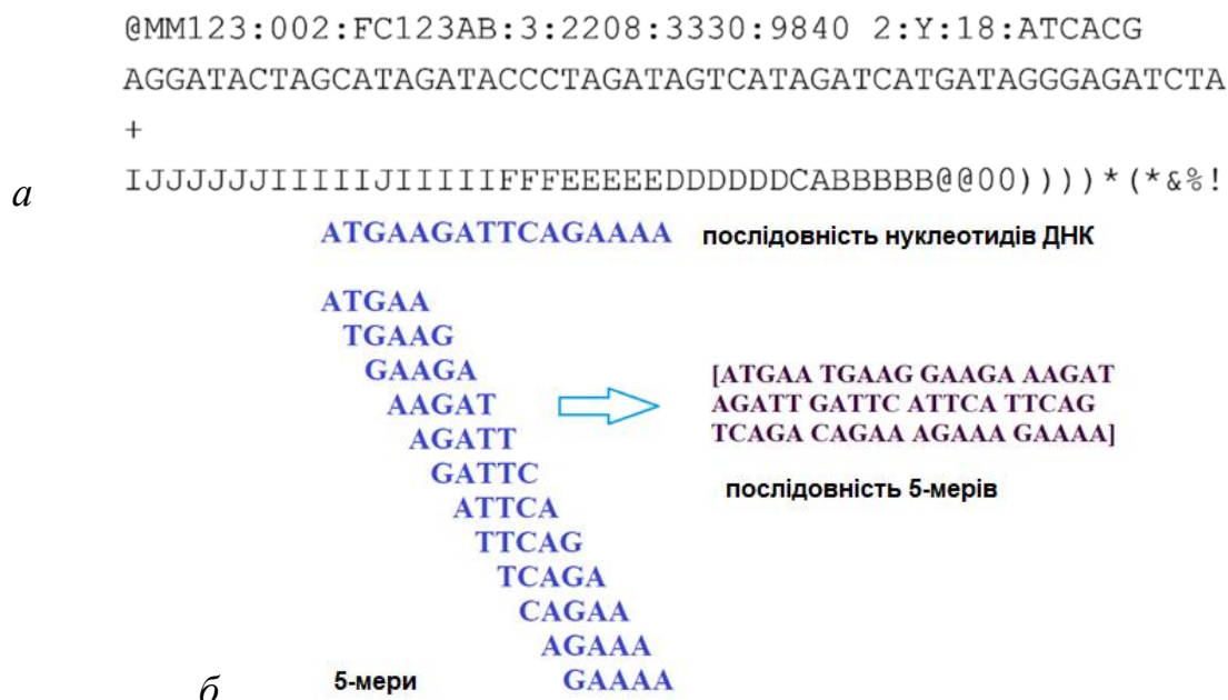
Рис.1 – Приклад фрагменту даних формату FASTQ (а) та отримання послідовності 4-мерів (б)
