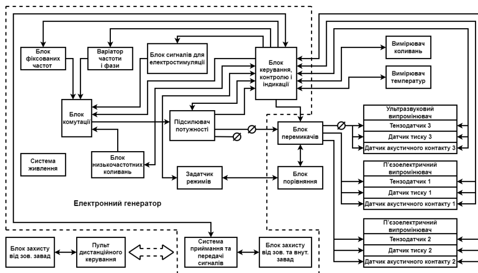
Рис. 1 – Структурна схема високоточної ультразвукової комп’ютерно-інтегрованої медичної системи
