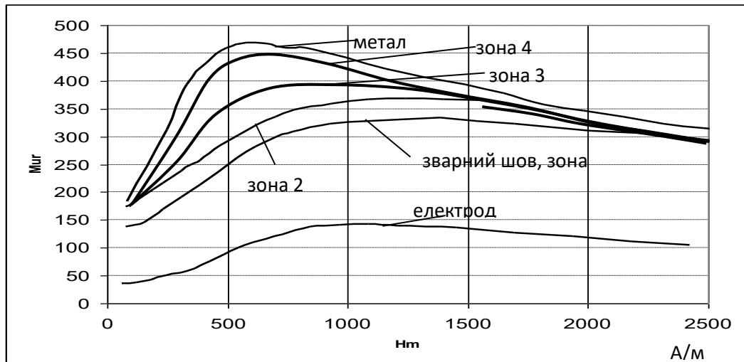
Рис. 2 – Магнітні характеристики матеріалу зварного шва, електрода та навколо шовної зони
