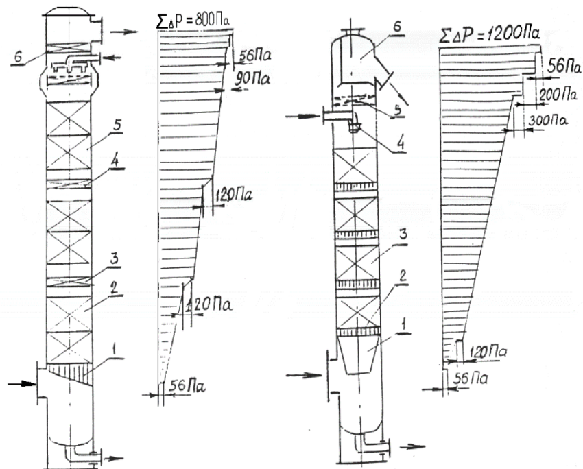
Рис.1. Епюри втрат напору в скруберах з регулярними листовими насадками (а- плоскопаралельною; б - Z - подібною ).
