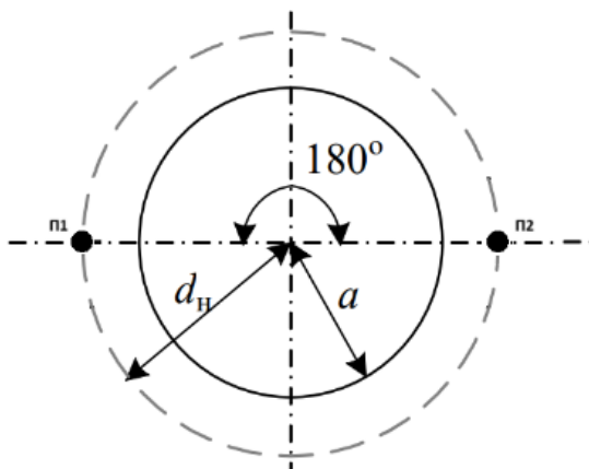
Рис. 1 – паралельне розташування провідників П1 та П2 з однаковим струмом
