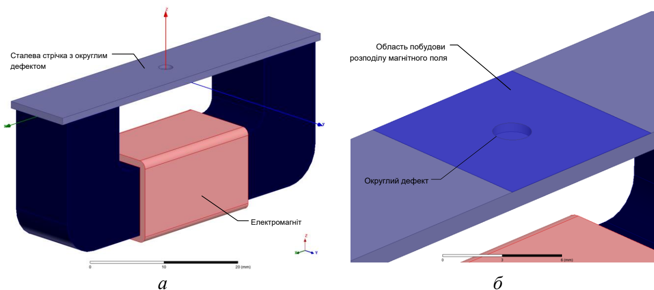
Рис. 1 – Система магнетизації сталевій стрічки : а – ескіз моделі; б – округлий дефект стрічки
