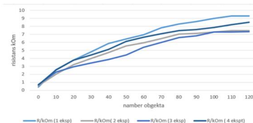
Рис. 2 – Графік зміни імпедансу біологічної тканини чотирьох об'єктів
