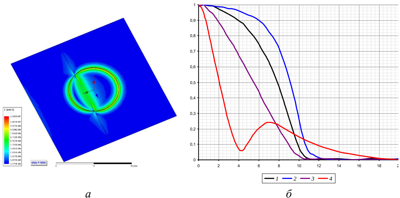
Рис. 2 – Результати моделювання: а – розподіл щільності вихрових струмів для круглого ВСП; б – сигнали ВСП при різній позиції дефекту
