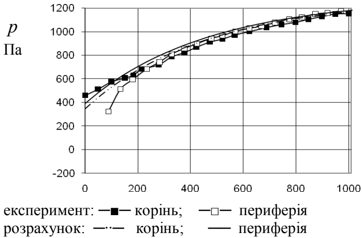
Рисунок 4 – Розподіл статичного тиску вздовж обводів дифузора
