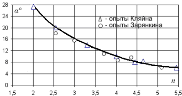
Рисунок 5 – Крива Кляйна
