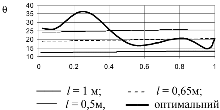
Рисунок 7 – Характер зміни кута \theta
