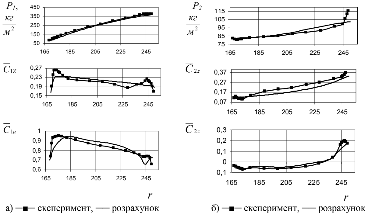
Рисунок 1 – Розподіл параметрів потоку
