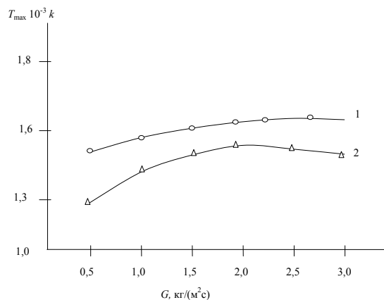
Рис. 3. Зависимость T_{max} от G , 1 – Al 2 O 3 , 2 – шамот.
