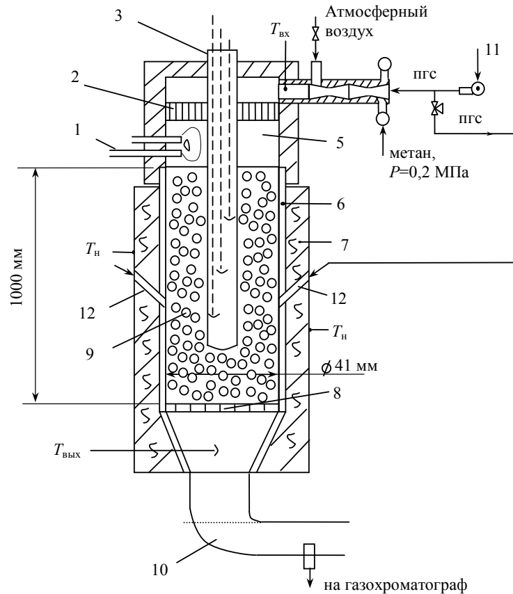
Рис. 1. Схема реактора:
