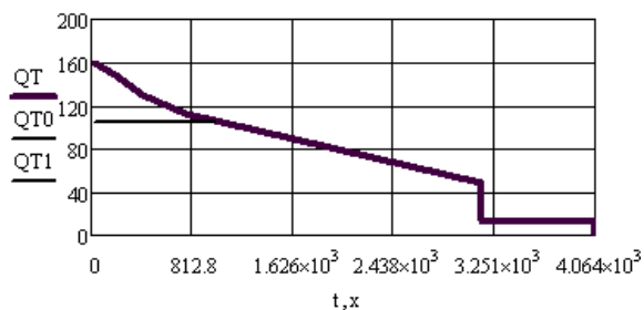
Рис. 2 – Графік річного відпуску теплоти теплофікаційною установкою в залежності від числа годин стояння температури зовнішнього повітря: QT – теплове навантаження, МВт; QT0 – теплове навантаження початкового (порівнювального) варіанту з відпуском теплоти Q_m = 105 МВт з наступним зниженням теплового навантаження у відповідності з графіком річного відпуску теплоти в діапазоні температур зовнішнього повітря від мінус 23 до плюс 8 ^{\circ}C при постійному нагріві \Delta t та змінній витраті G_{мв} мережної води; QT0I – теплове навантаження першого варіанту з відпуском теплоти Q_m = 105 МВт (90 Гкал/год) та наступним зниженням у відповідності з графіком річних витрат теплоти в діапазоні температур зовнішнього повітря від мінус 23 до плюс 8 ^{\circ}C при постійних температурі прямої мережної води t_1 та витраті G_{мв} мережної води
