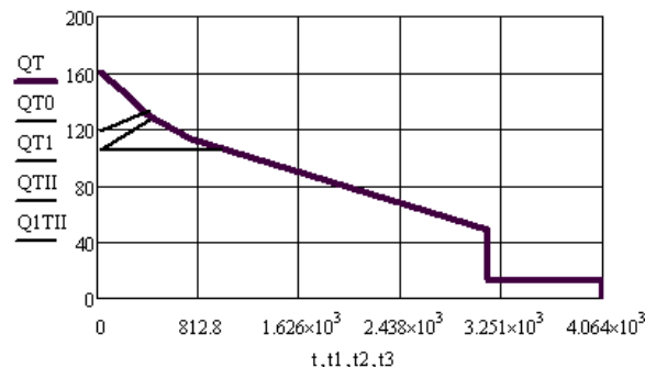
Рис. 3 – Графік річного та додаткового відпуску теплоти теплофікаційною установкою з забезпеченням постійних температур прямої мережної води t_{11} = 156 та t_{12} = 168 ^{\circ}C : QTII – теплове навантаження додаткового відпуску теплоти теплофікаційною установкою з забезпеченням постійної температури прямої мережної води t_{11} = 156 ^{\circ}C ; QTIII – теплове навантаження додаткового відпуску теплоти теплофікаційною установкою з забезпеченням постійної температури прямої мережної води t_{12} = 168 ^{\circ}C
