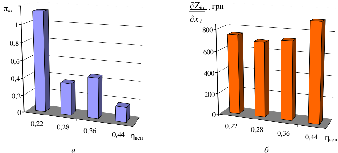
Рис. 1 – Анализ термoeкономических показателей чувствительности структурной схемы ХМ при варьировании \bar{\eta}_{\text{исп}} :
