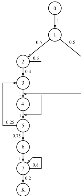
Рисунок 1.3 – Мінімізований граф алгоритму
