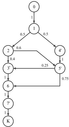
Рисунок 1.5 – Граф алгоритму без циклів
