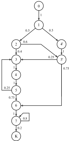
Рисунок 1.4 – Еквівалентний граф алгоритму
