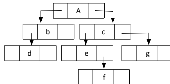
Рисунок 8.2 – Двійкове дерево
