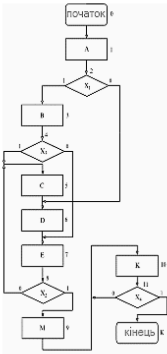
Рисунок 1.1 – Схема алгоритму
