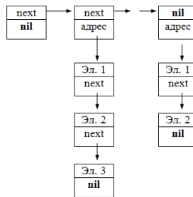
Рисунок 8.1 – Список списків
